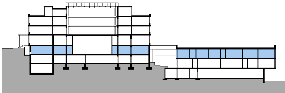
Schnitt Coupe
