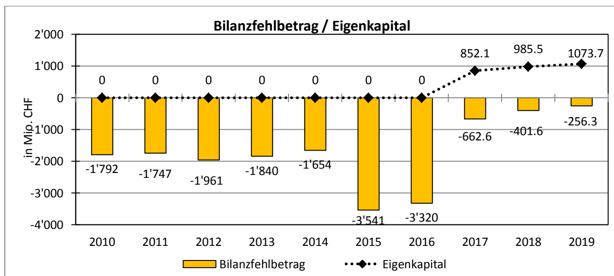
Abbildung 6: Bilanzfehlbetrag / Eigenkapital, 2010 – 2019
