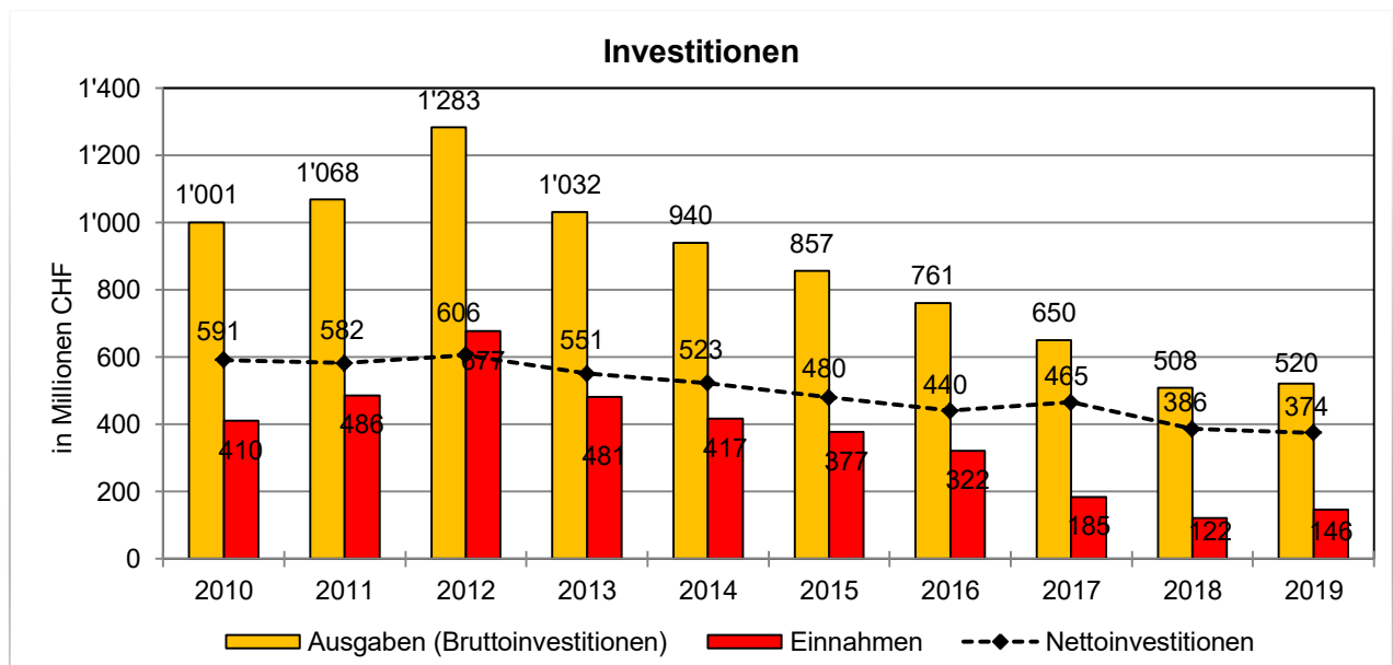
Abbildung 5: Investitionsrechnung, 2010 – 2019
