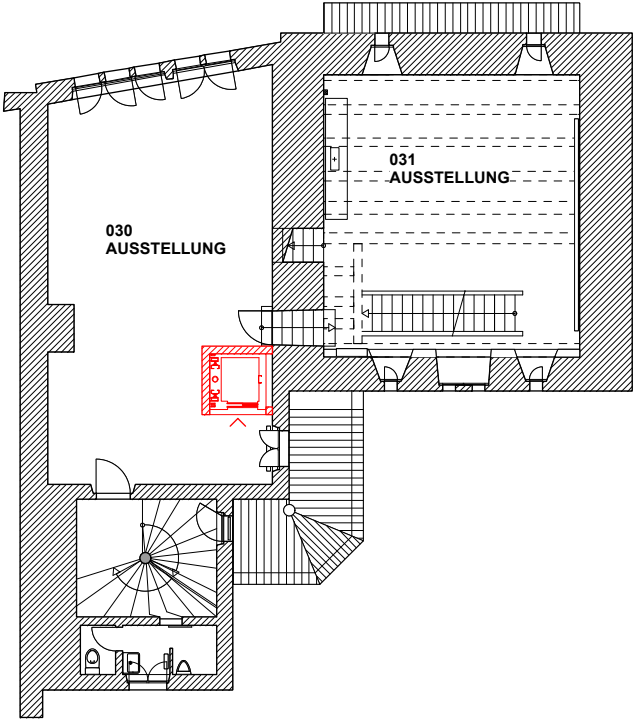
3. OBERGESCHOSS
