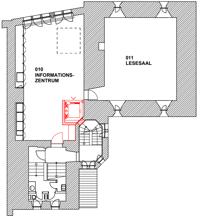
1. OBERGESCHOSS
