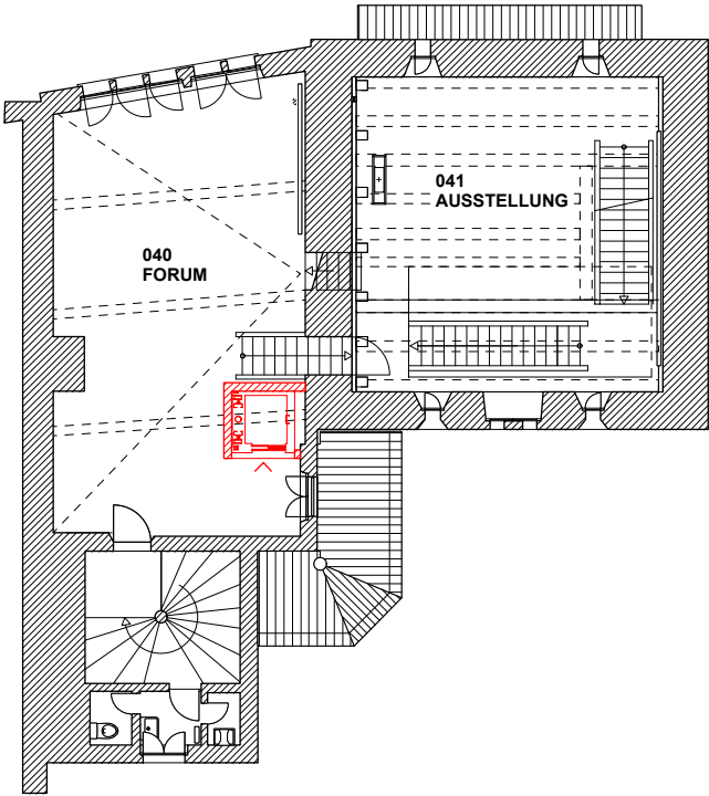
4. OBERGESCHOSS
