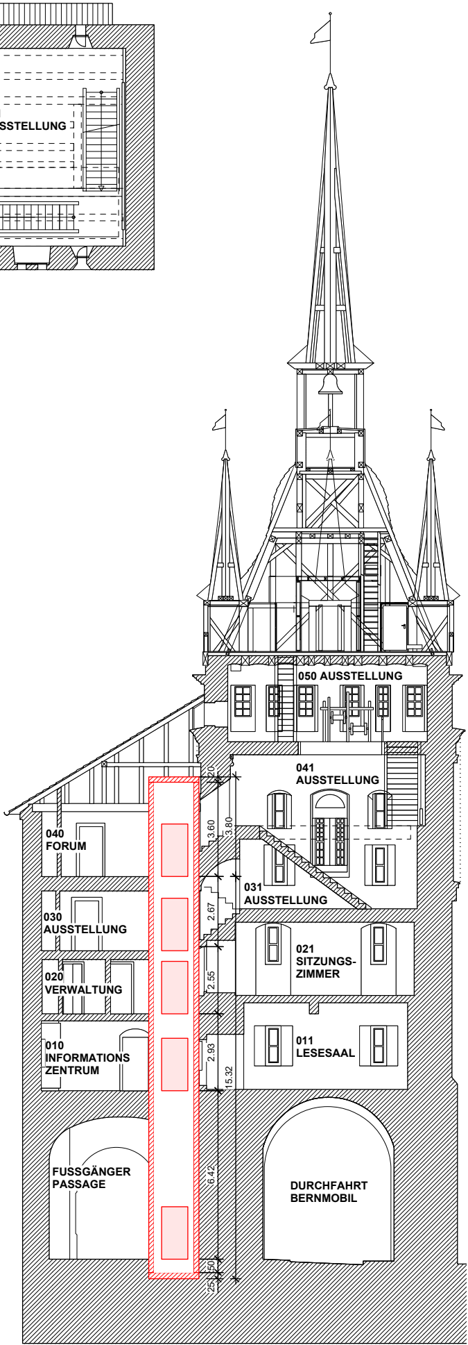
SCHNITT
