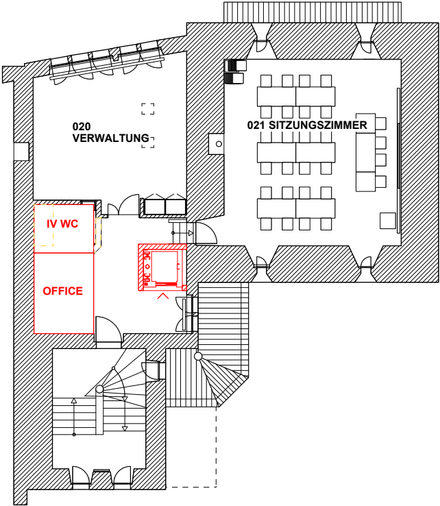
2. OBERGESCHOSS
