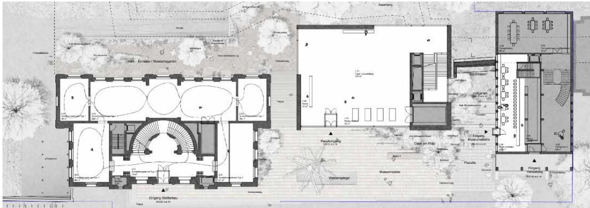
Abbildung aus dem Jurybericht: Grundriss Erdgeschoss
