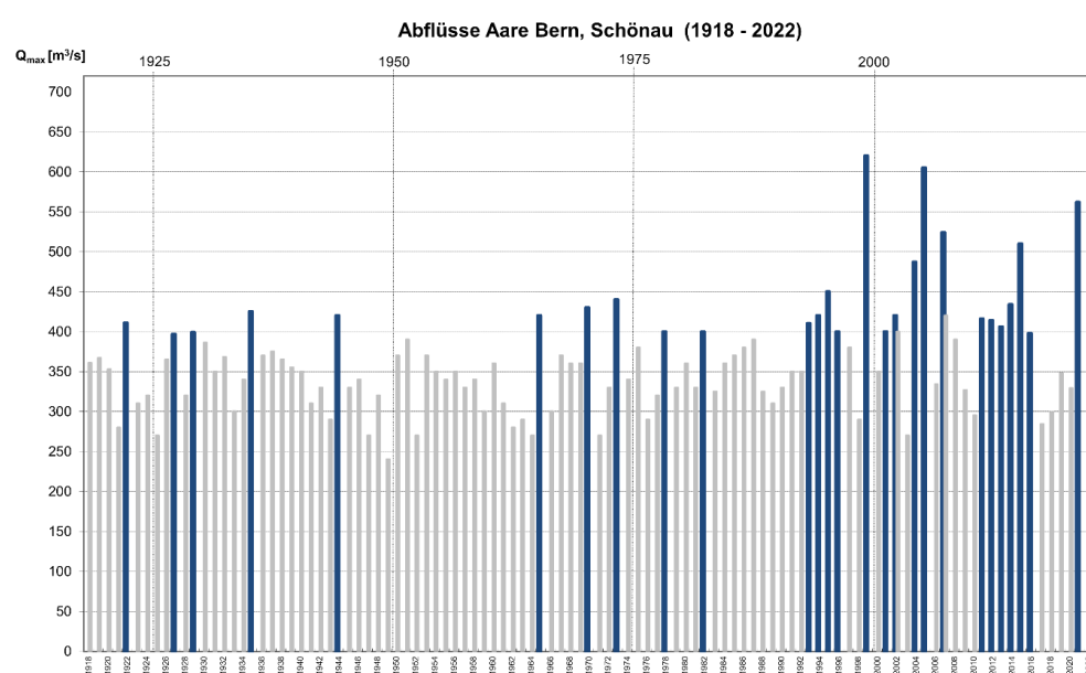
Abbildung 2: Maximale jährliche Abflussmengen bei der Messtelle Schönau.
